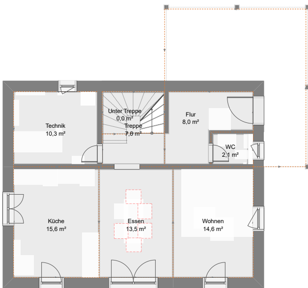
GRUNDRISS ERDGESCHOSS
