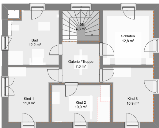
GRUNDRISS OBERGESCHOSS
